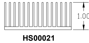
Longitudinal Heatsinks
