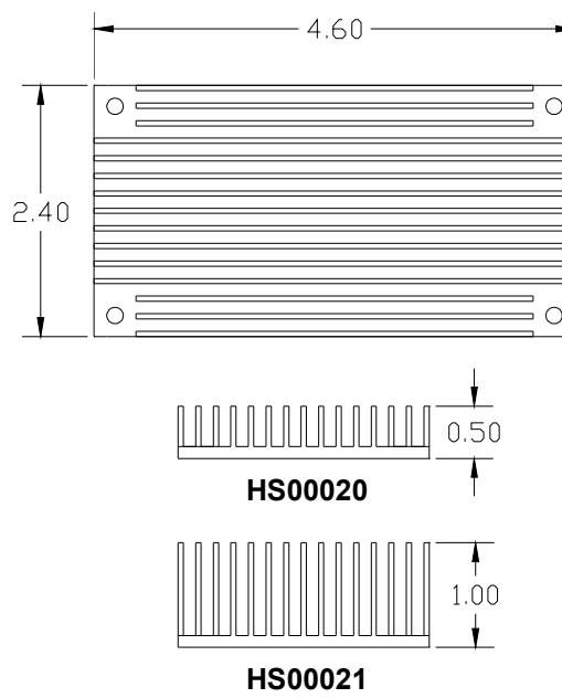
Longitudinal Heatsinks
